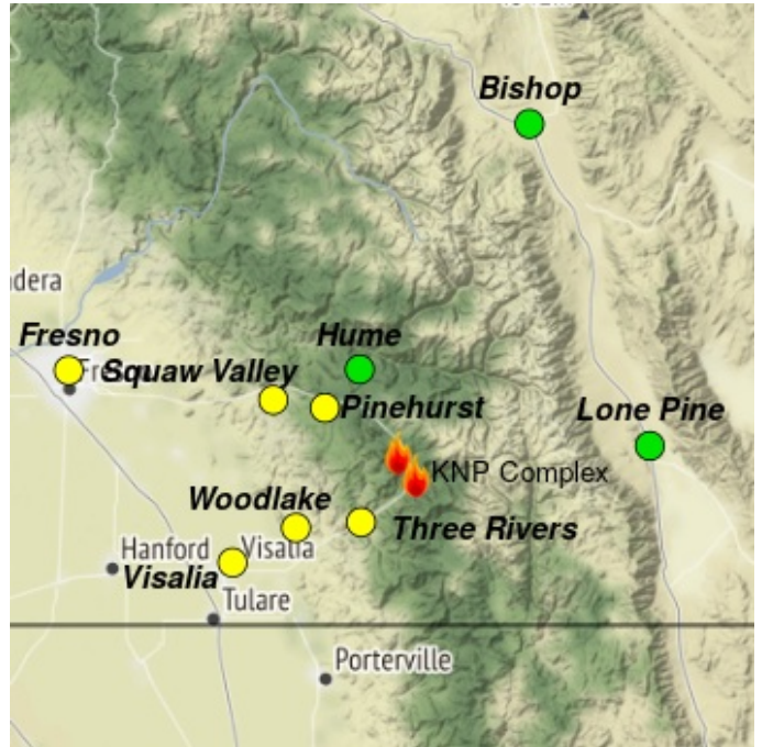
Pronóstico del ICA* para 14 de octubre de 2021
